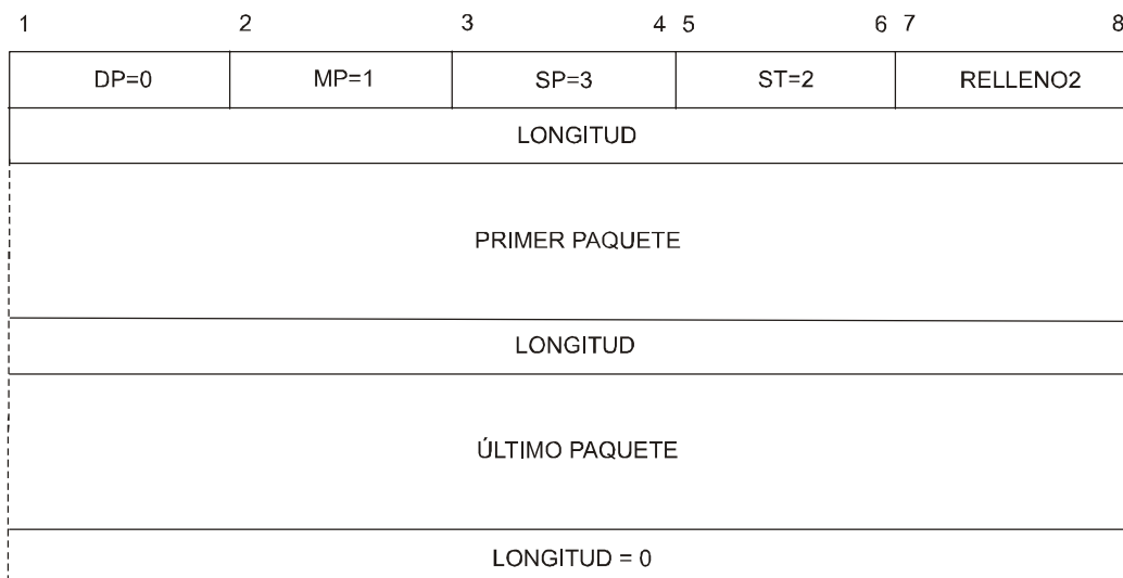
Figura 5-20. Paquete de MULTIPLEX
