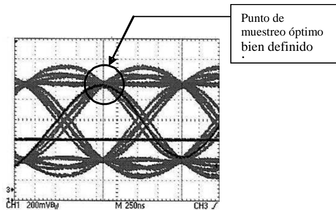
Figura 12-3. Diagrama en ojo ideal
