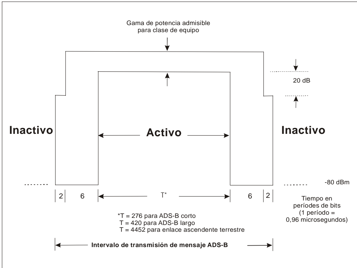
Figura 12-2. Perfil de tiempo/amplitud de la transmisión de mensajes UAT
