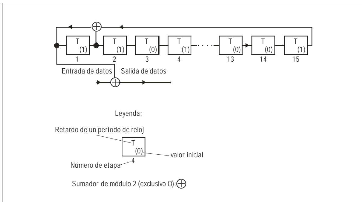
Figura 6-2. Generador PN de secuencia de codificación secreta de bits
