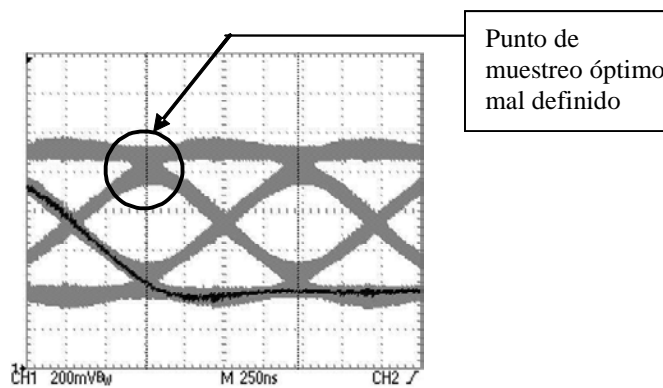
Figura 12-4. Diagrama en ojo con distorsión
