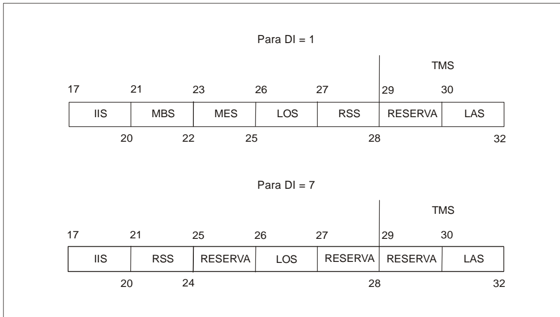
Figura 5-1. Estructura del campo SD
