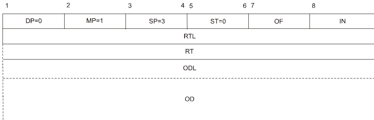
Figura 5-19. Paquete de RUTA
