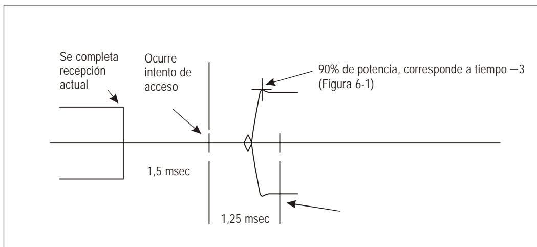
Figura 6-3. Tiempo de actuación de recepción a transmisión
