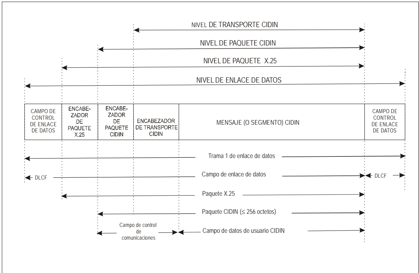
Figura 8-2. Terminología de la CIDIN
