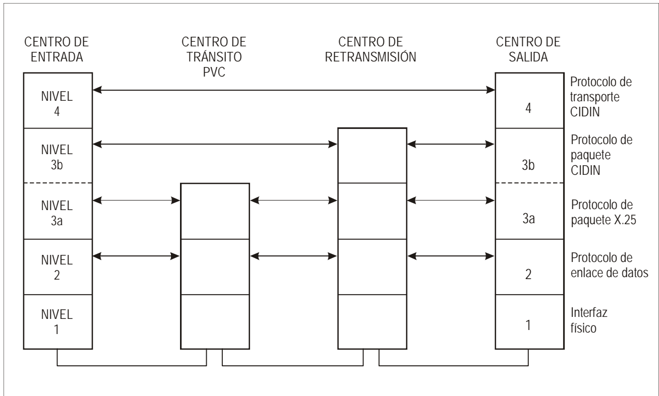
Figura 8-1. Niveles de protocolo CIDIN
