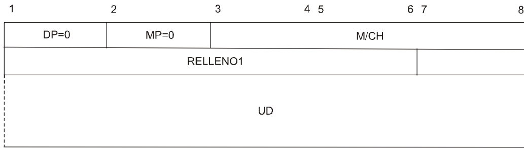
Figura 5-21. Paquete de MSP FORMA CORTA
