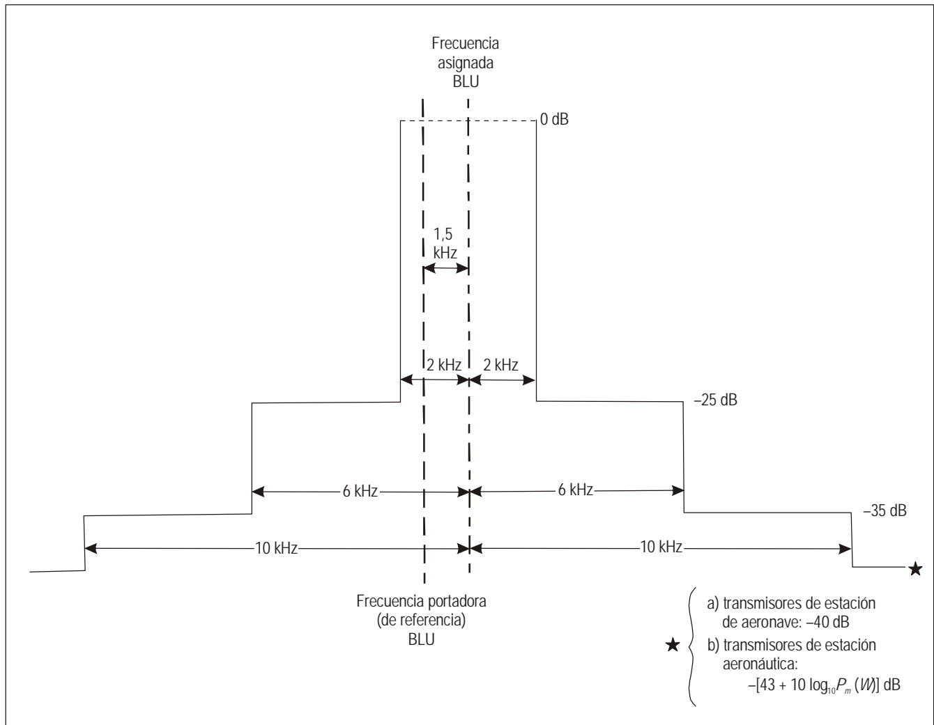
Figura 2-1. Límites del espectro requeridos (en cuanto a la potencia media) para los tipos de transmisores de estaciones de aeronaves y para los transmisores de estaciones aeronáuticas instalados inicialmente antes del 1 de febrero de 1983
