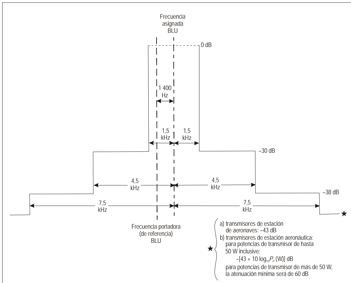
Figura 2-2. Límites del espectro requeridos (en cuanto a la potencia máxima) para los transmisores de estaciones de aeronaves instalados inicialmente después del 1 de febrero de 1983 y para los transmisores de estaciones aeronáuticas que se utilicen después del 1 de febrero de 1983
