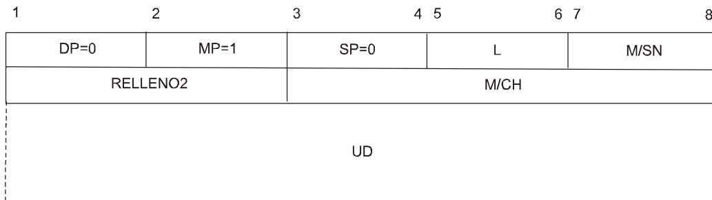
Figura 5-22. Paquete de MSP FORMA LARGA
