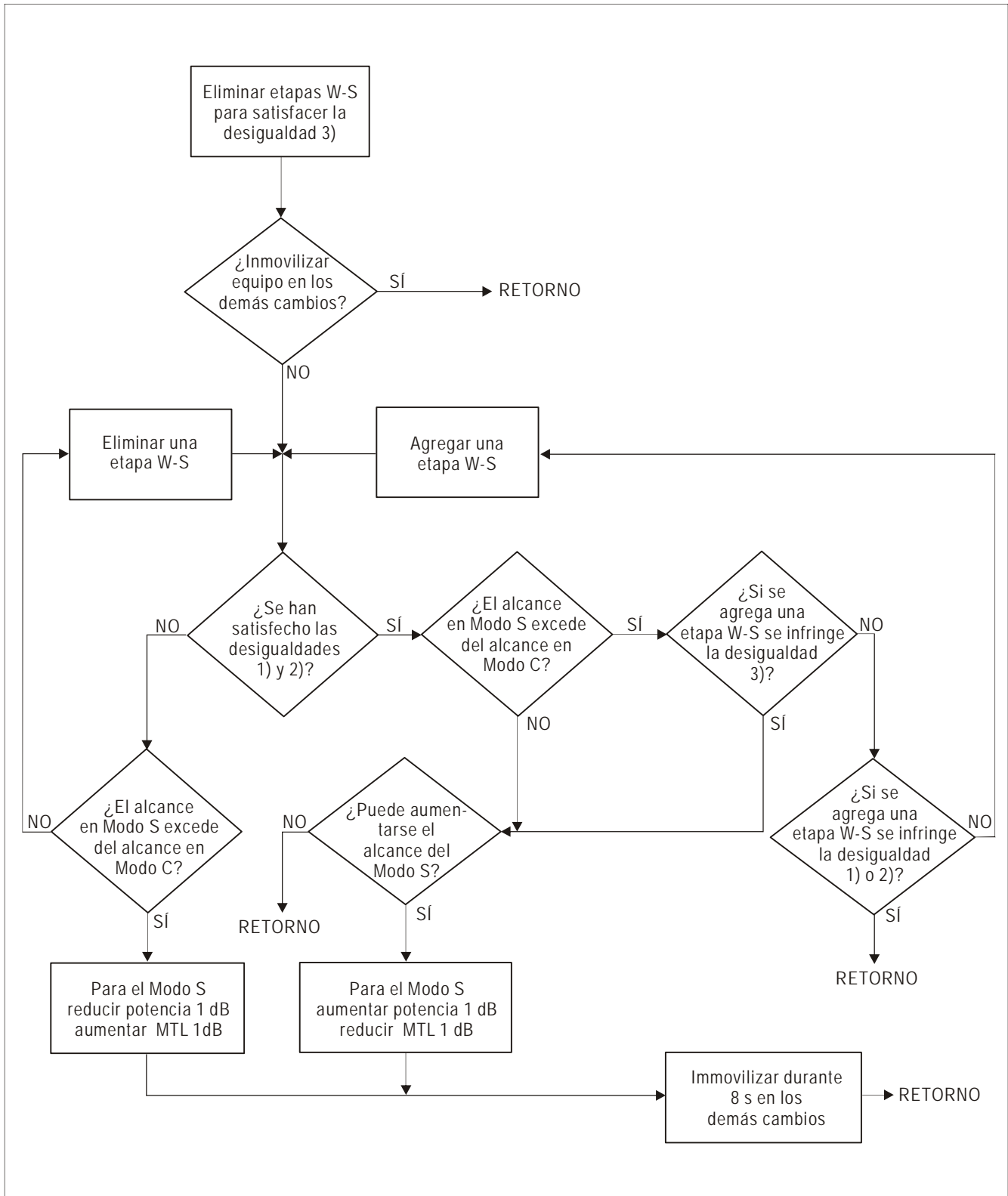
Figura A-4. Diagrama de limitación de interferencias
