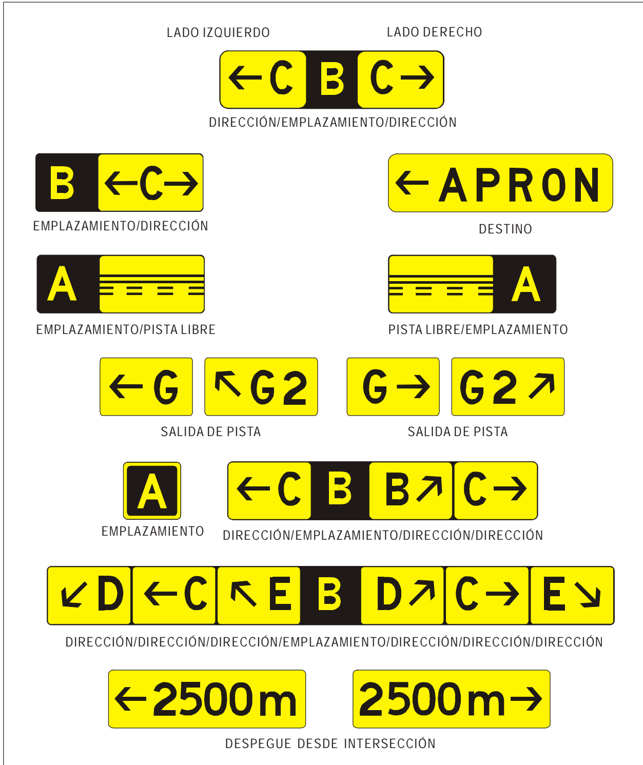
Figura 5-29. Letreros de información
