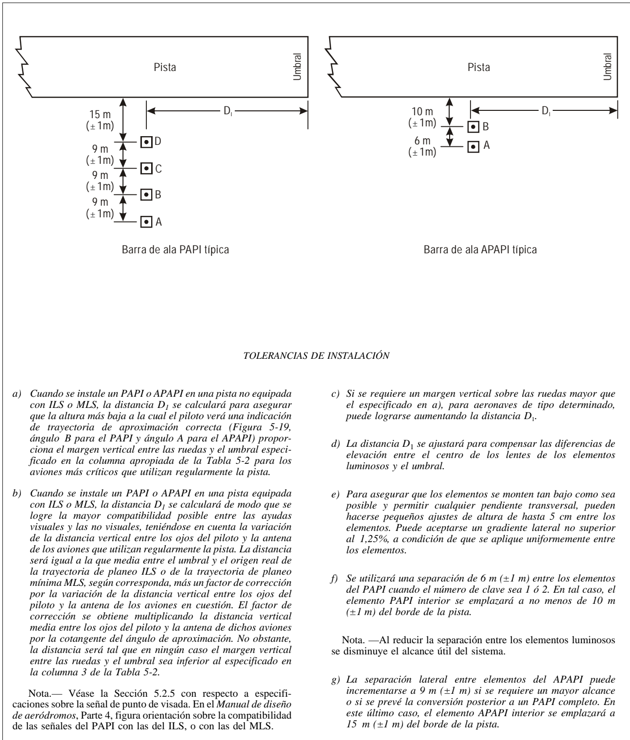
Figura 5-18. Emplazamientos del PAPI y del APAPI
