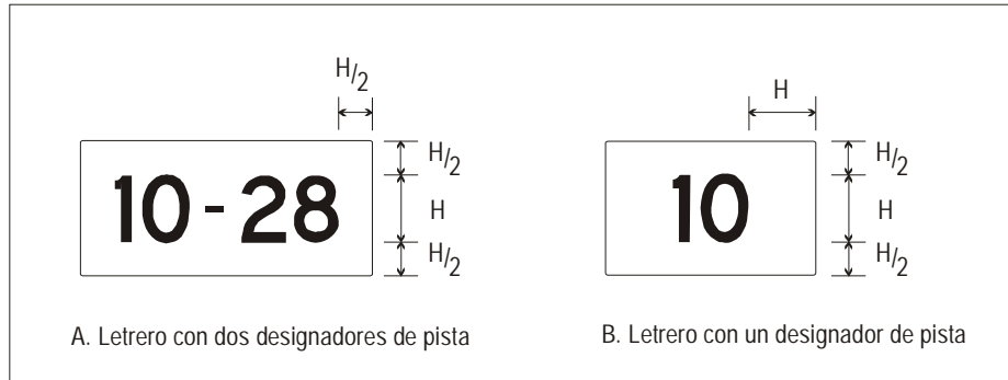
Figura A4-3. Dimensiones de los letreros
