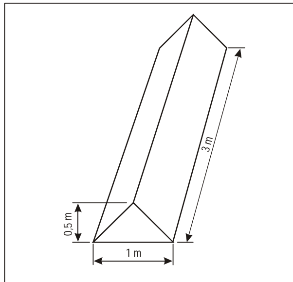
Figura 5-32. Balizas delimitadoras
