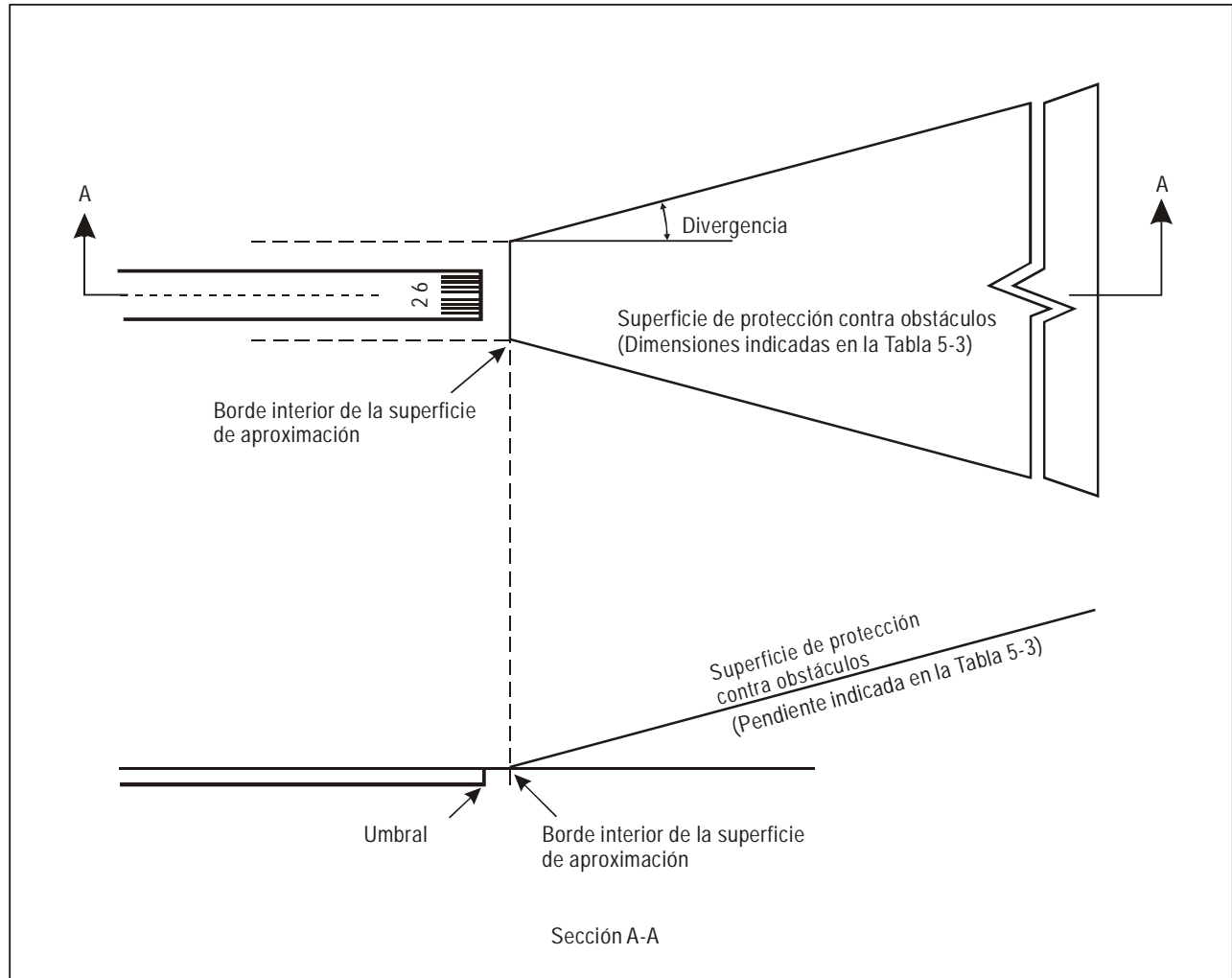
Figura 5-20. Superficie de protección contra obstáculos para los sistemas visuales indicadores de pendiente de aproximación
