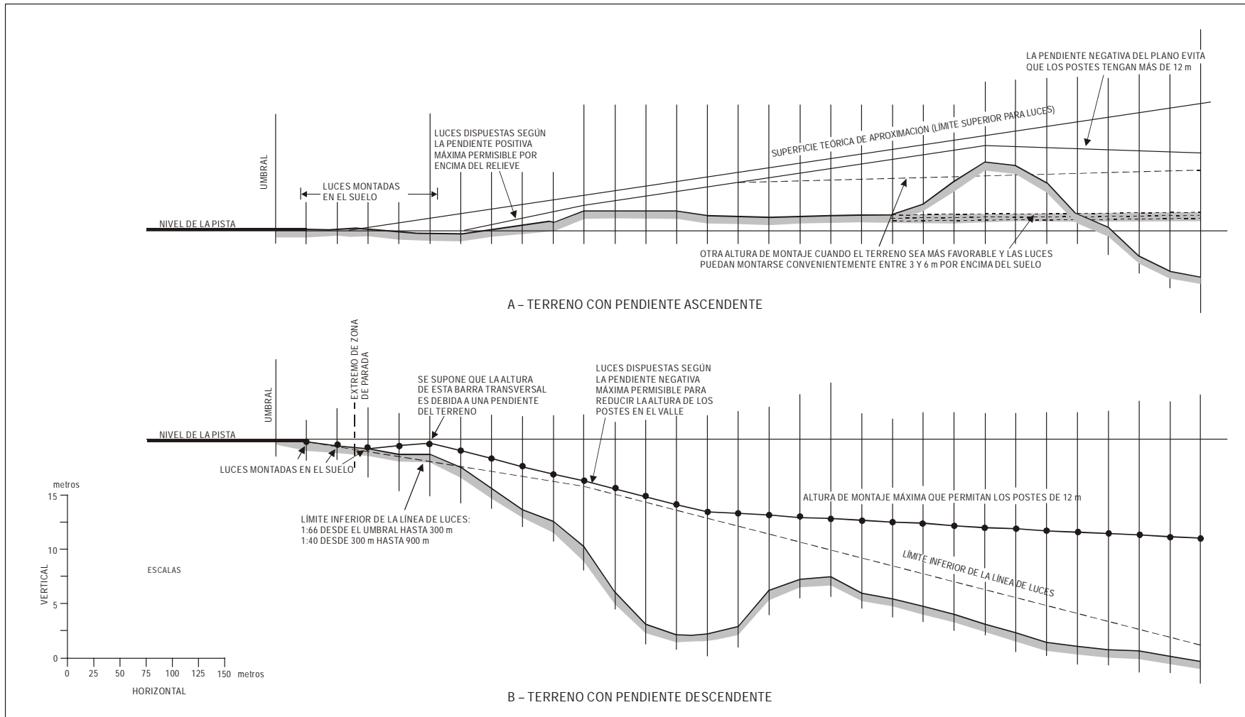
Figura A-7. Tolerancias verticales de instalación
