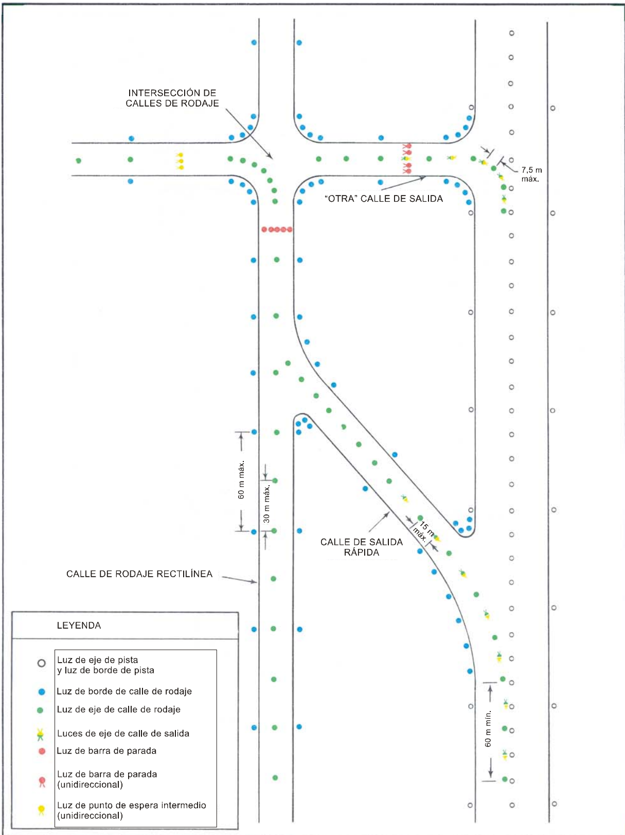
Figura 5-24. Iluminación de calles de rodaje
