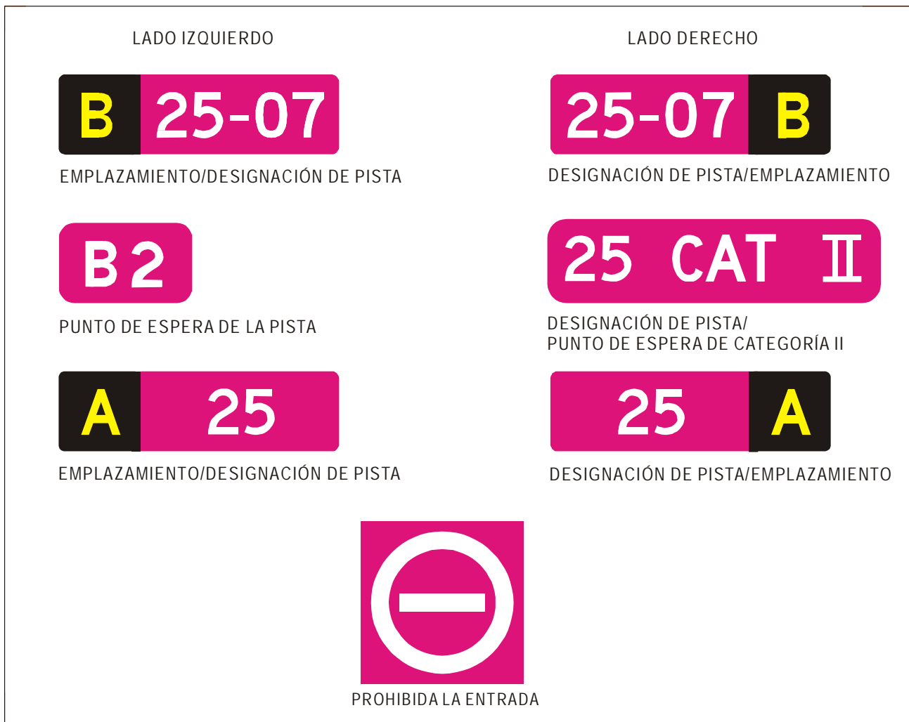
Figura 5-28. Letreros con instrucciones obligatorias
