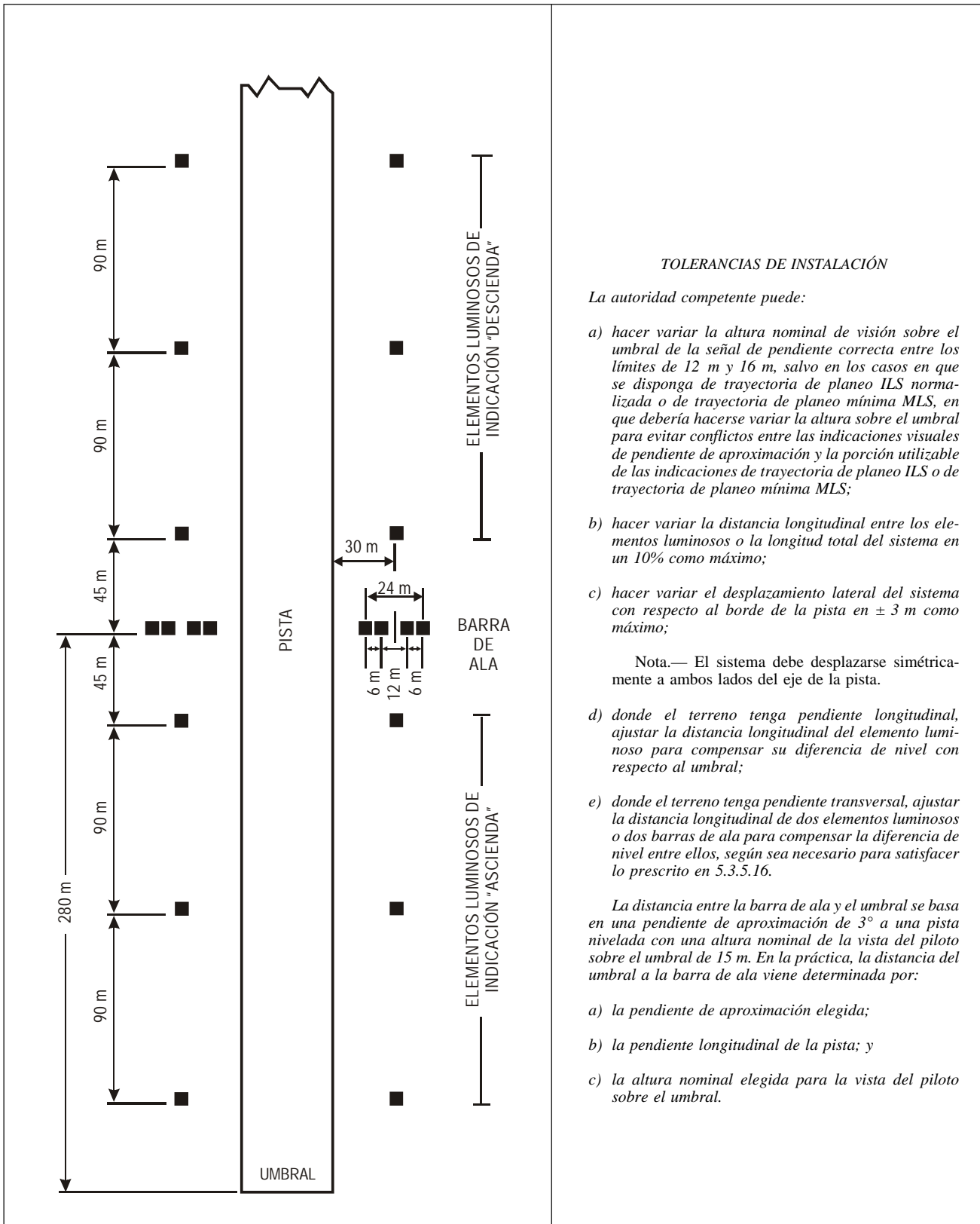
Figura 5-16. Emplazamiento de los elementos luminosos del T-VASIS
