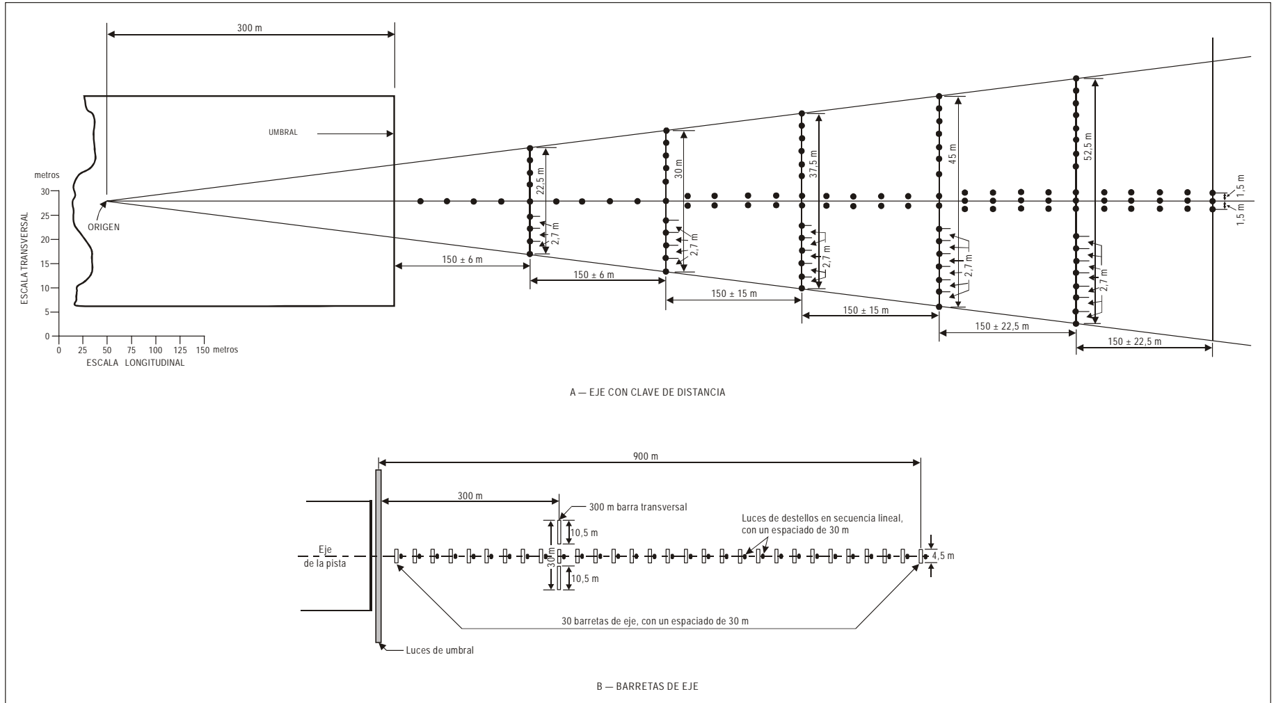
Figura A-6. Sistemas de iluminación de aproximación de precisión de Categoría I
