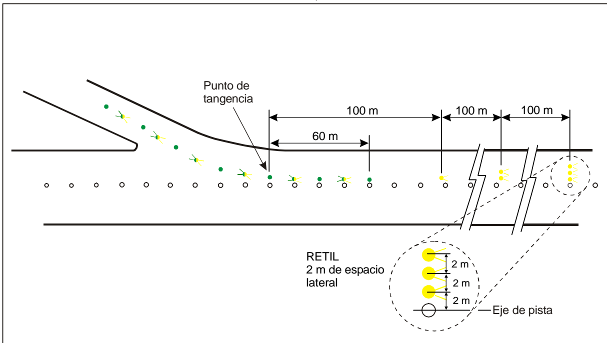
Figura 5-23. Luces indicadoras de calle de salida rápida
