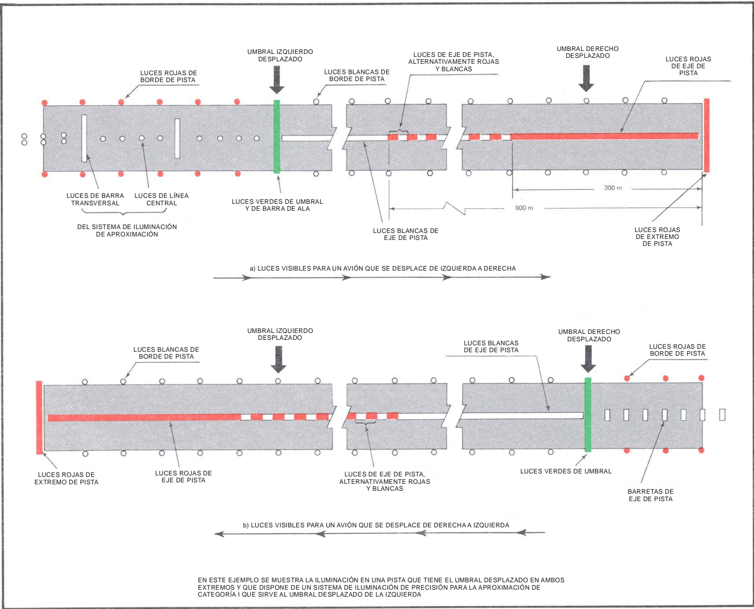
Figura 5-22. Ejemplo de iluminación de aproximación y de la pista en las pistas con umbrales desplazados
