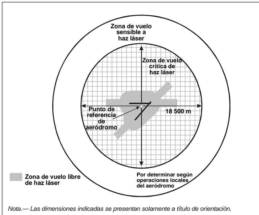
Figura 5-10. Zonas de vuelo protegidas
