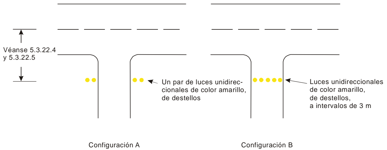
Figura 5-27. Luces de protección de pista
