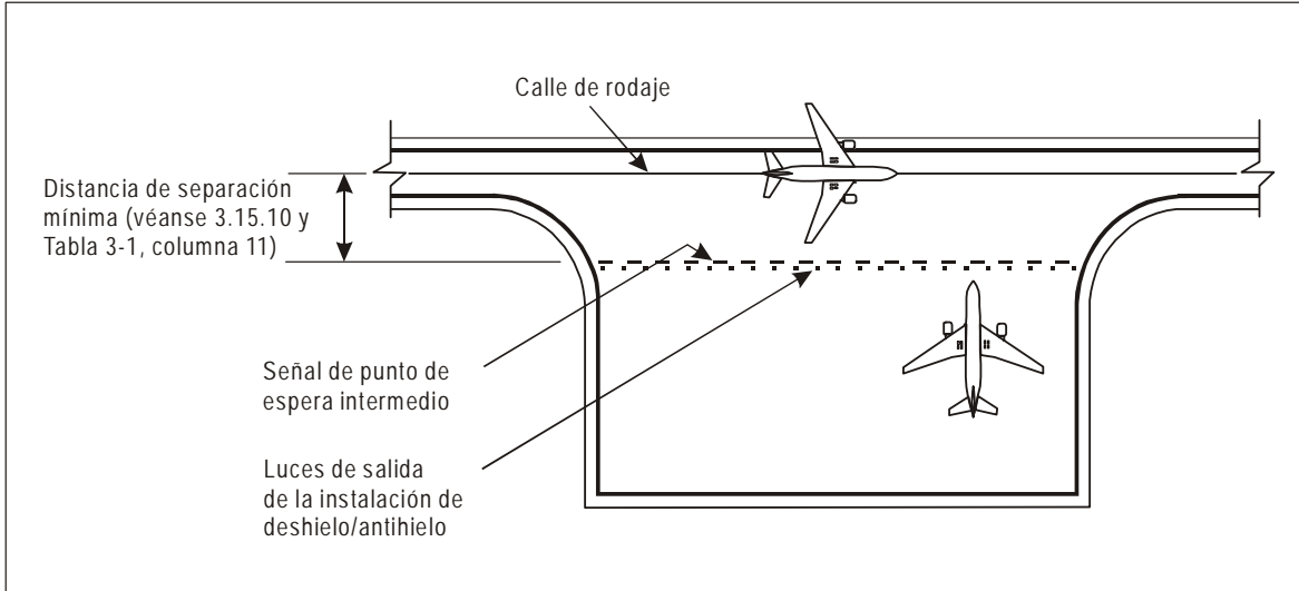
Figura 5-26. Típica instalación de deshielo/antihielo distante
