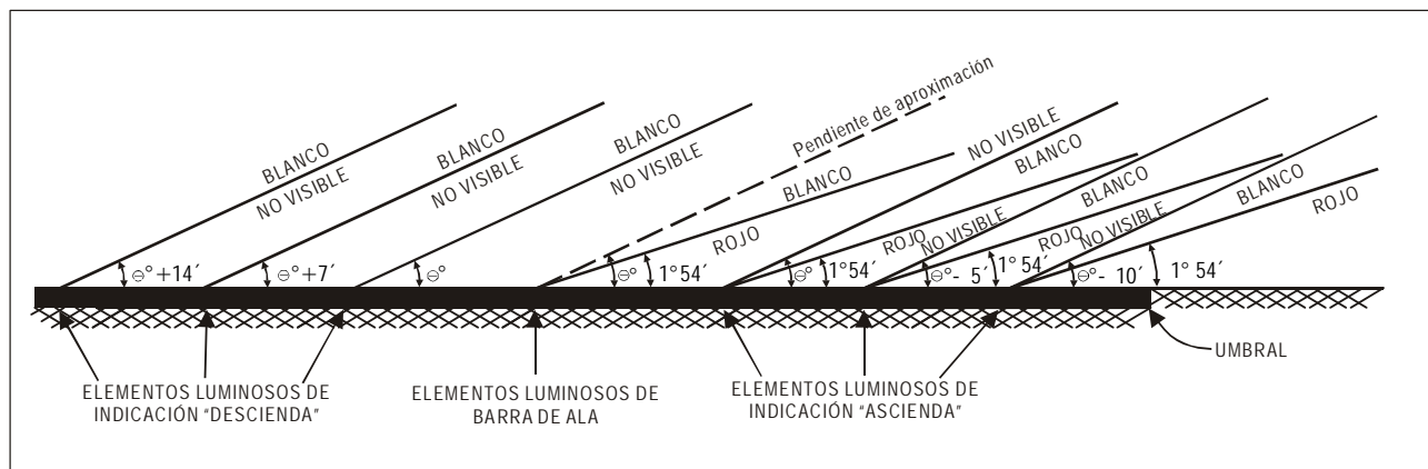
Figura 5-17. Haces luminosos y reglaje del ángulo de elevación del T-VASIS y del AT-VASIS
